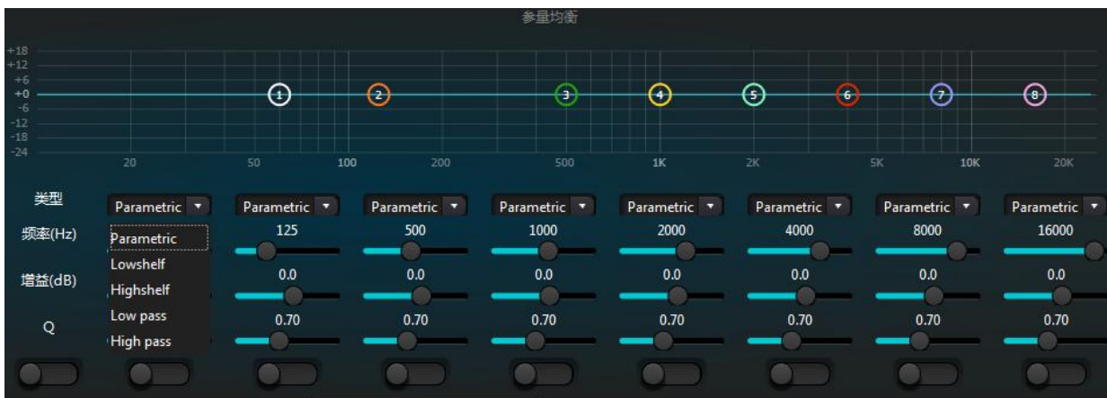
图 3.6 均衡器
